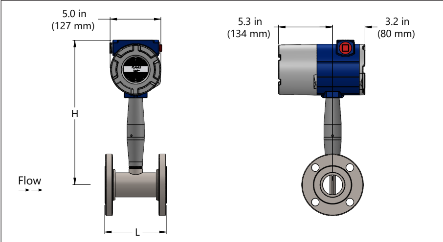
VF4 Inline Flanged
